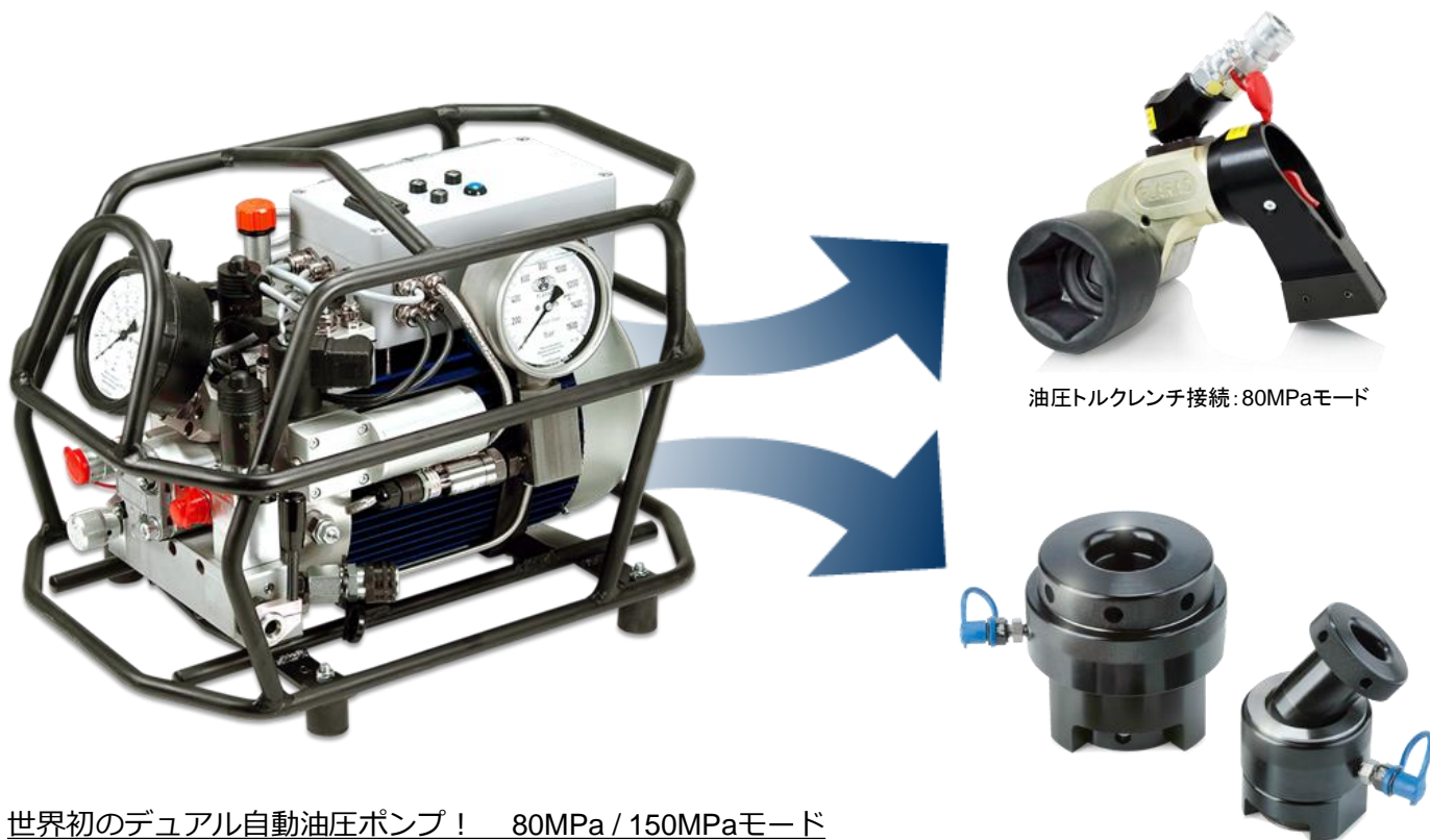
ボルトテンショナー接続: 150MPaモード
